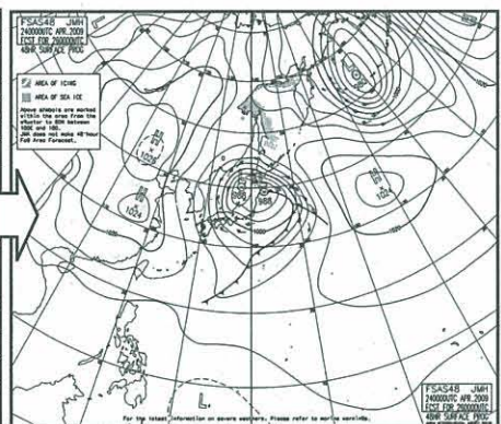
48時間後の予想天気図
