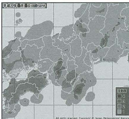
雷ナウキャスト
